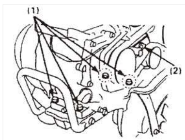
(1) Tornillos de montaje del motor (2) Tornillo de tensionado del motor
